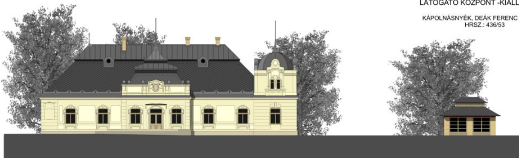
ÉK-1, BEJÁRATI HOMLOKZAT
